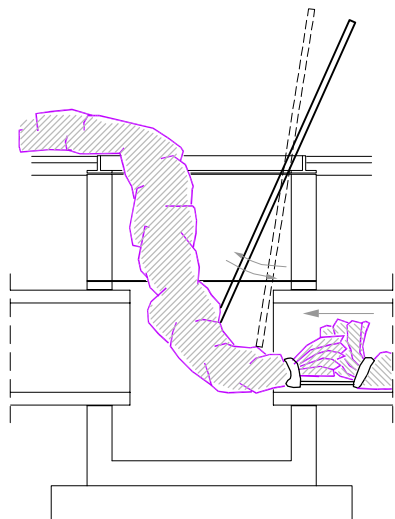
RIMOZIONE MANICHETTA (FASE DI RIMOZIONE MANICHETTA NELLA MANUTENZIONE STRAORDINARIA)
